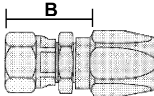
SAE 45° FLARE SWIVEL NON-MANDREL
